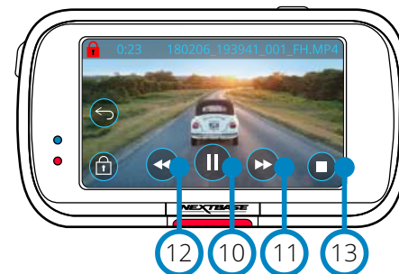
Video Prehrávanie
