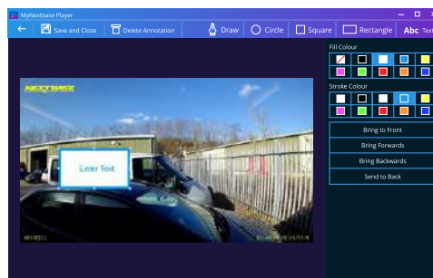
Anotáčne Okno
