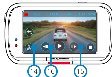
Video Zastavené
